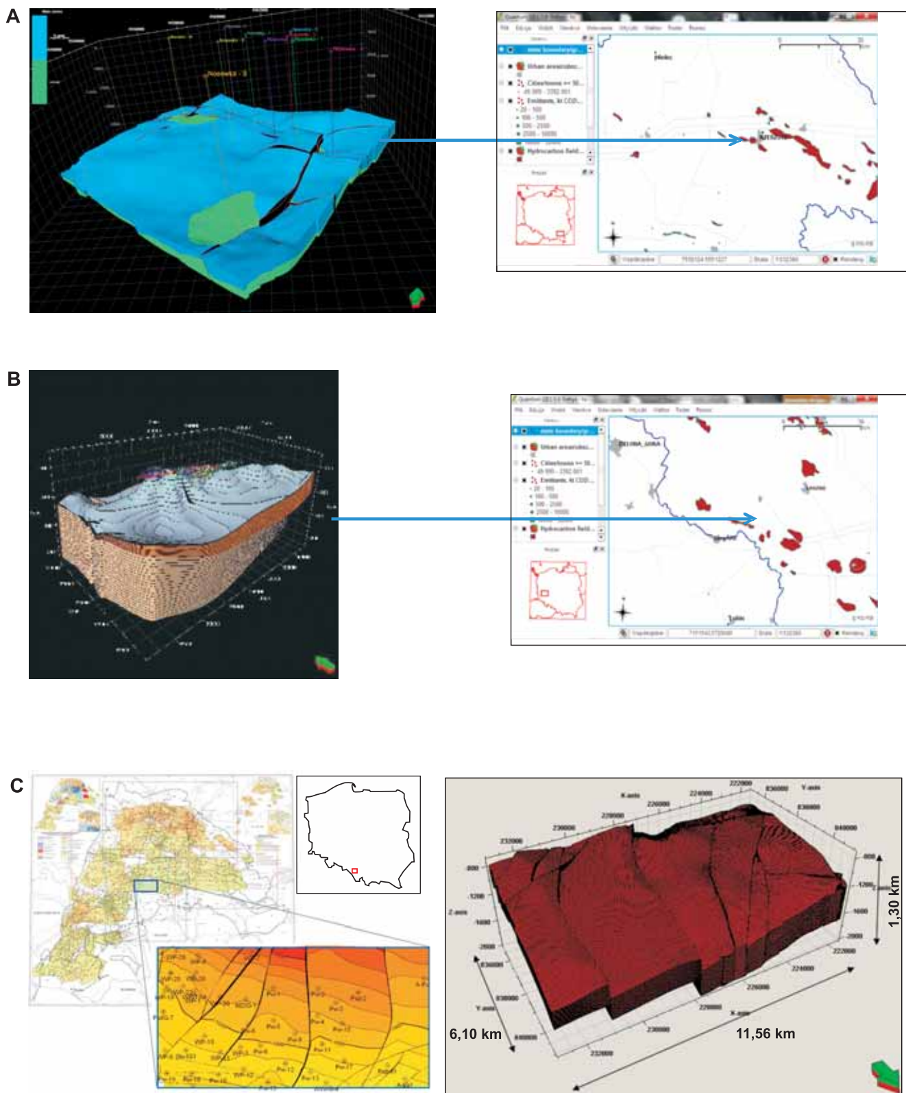
Fig. 5. A. Model złoża ropy Nosówka (prace pod kierunkiem W. Szotta (INiG)). B. Model złoża gazu Wilków (prace pod kierunkiem S. Nagy'a i B. Papiernika (AGH UST), raport niepublikowany). C. Model złoża metanu w pokładach węgla Warszawice-Pawłowice (prace pod kierunkiem J. Chećki (CMI) i J. Jureczki (PIG-PIB OG), raport niepublikowany)
